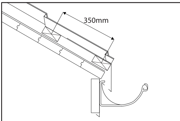
Rys. 8 Rozstaw łąt
