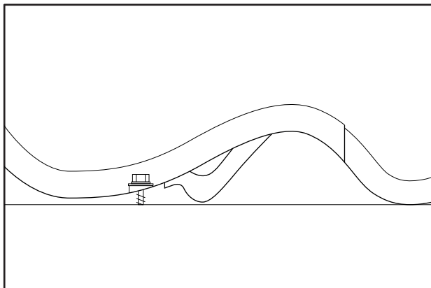
Rys. 10 Montaż arkuszy
